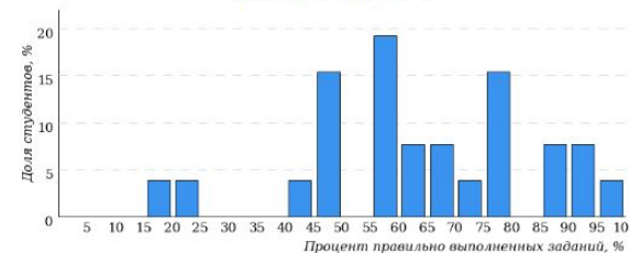
Гистограмма плотности распределения результатов тестирования
