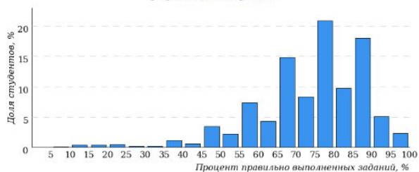
Гистограмма плотности распределения результатов тестирования
