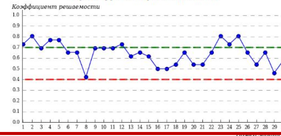
Карта коэффициентов решаемости заданий
