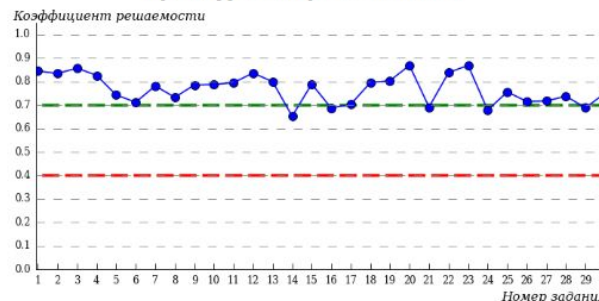
Карта коэффициентов решаемости заданий
