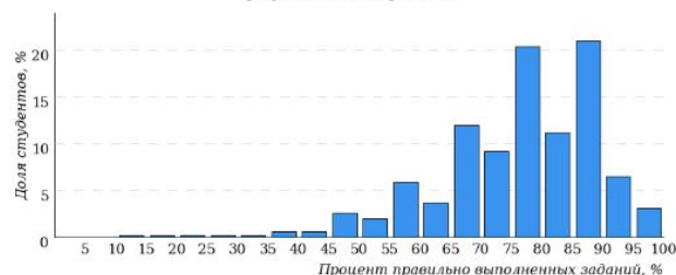
Гистограмма плотности распределения результатов тестирования
